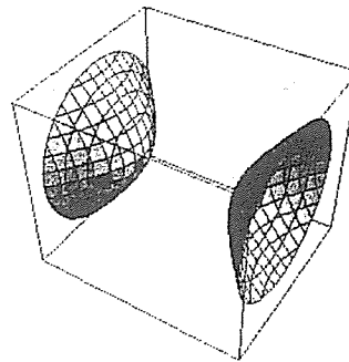
f) hiperboloide de dos hojas
